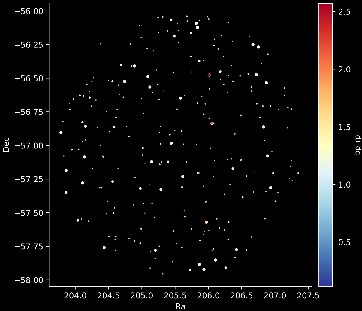
GALAH DR4 Field: [7224] Stars: 248
