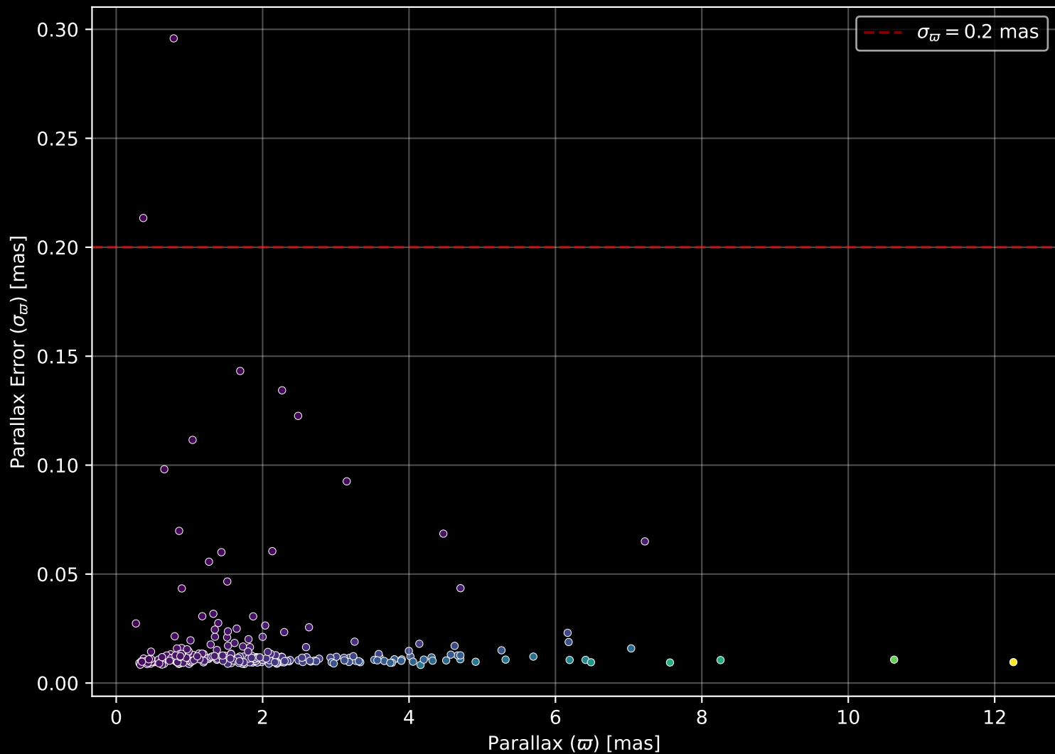
GALAH DR4 Field: [7224] Parallax Quality (n= 248)
