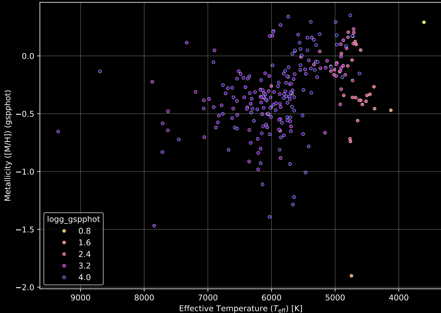
GALAH DR4 Field: [7224] Stellar Population Parameters (n= 248)
