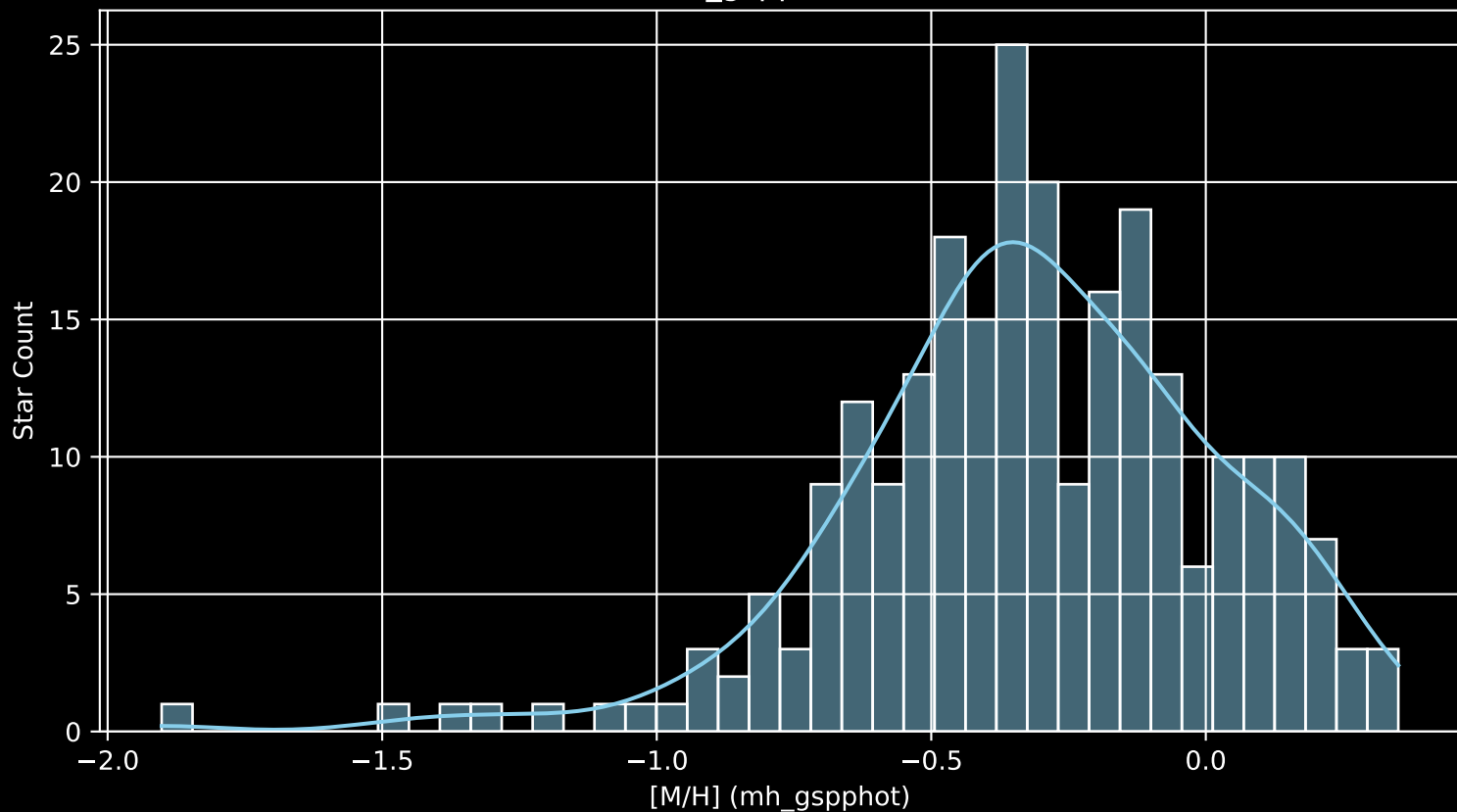
GALAH DR4 Field: [7224] [M/H] (mh_gspphot) (n= 248)
